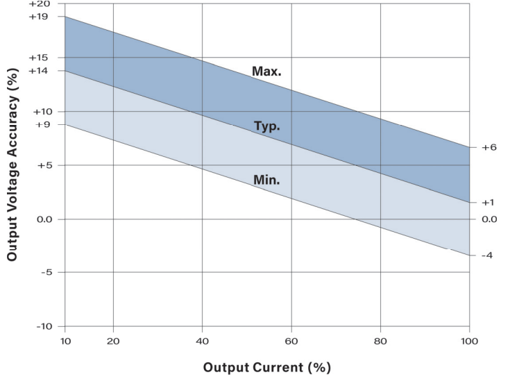
MIG215L-1509HI: -9V Output
