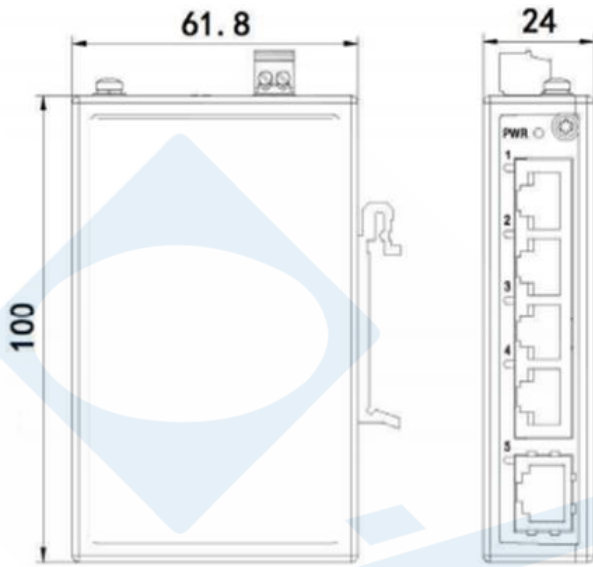
ISE2003D/2005D/5005D
