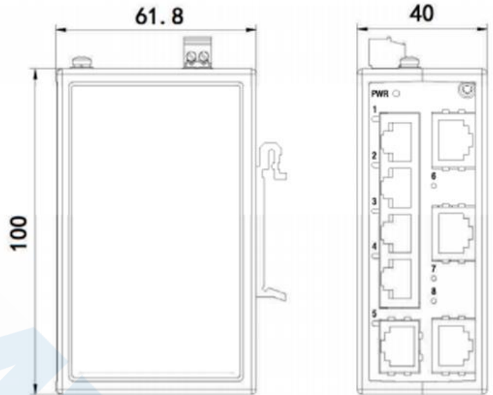
ISE2008/5008D
