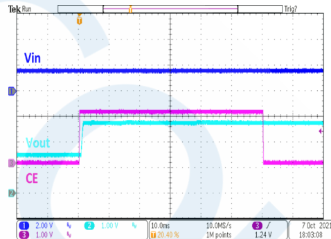
HT7727FA Chip Enable/Disable
