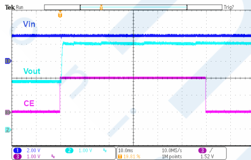
HT7750FA Chip Enable/Disable
