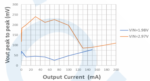
HT7733FA Ripple @L=10µH Cout=10µF
