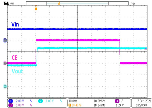
HT7733FA Chip Enable/Disable
